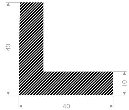
225.00.101 EPDM 15° Shore zwart rollengte 25 meter
